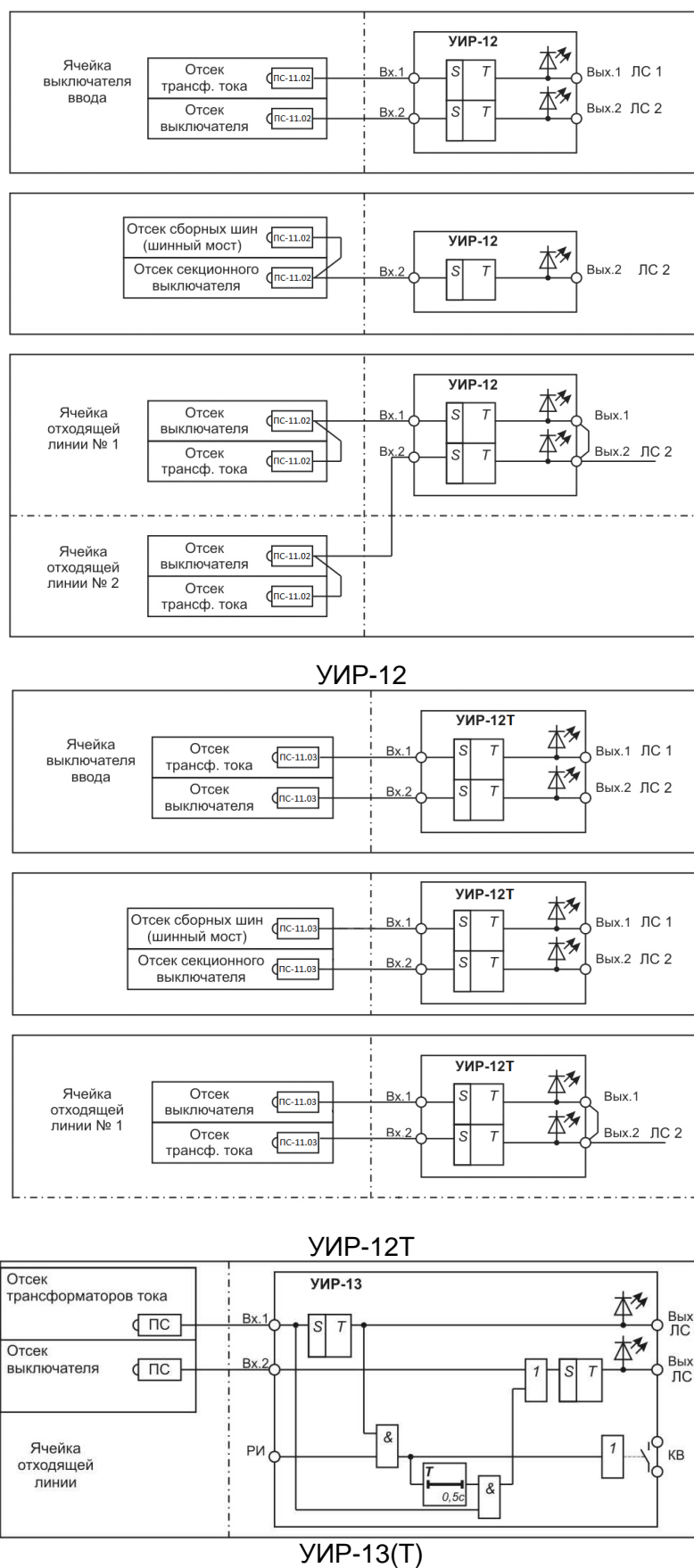
Рисунок В.1 – Логика работы УИР
