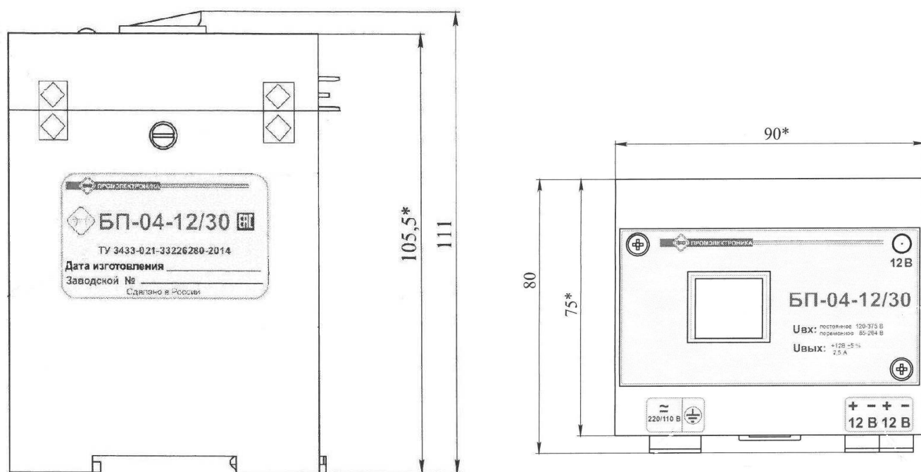
Рисунок Г.11 – Габаритные размеры БП-04-12/30
