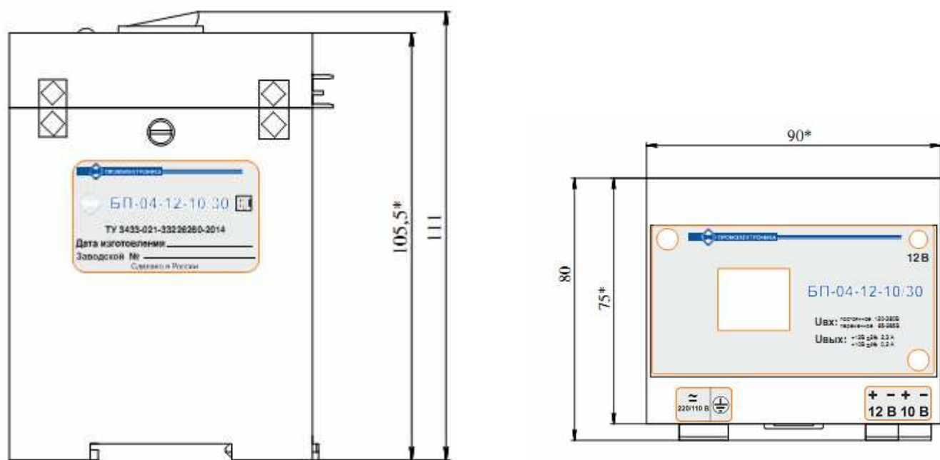
Рисунок Г.12 – Габаритные размеры БП-04-12-10/30
