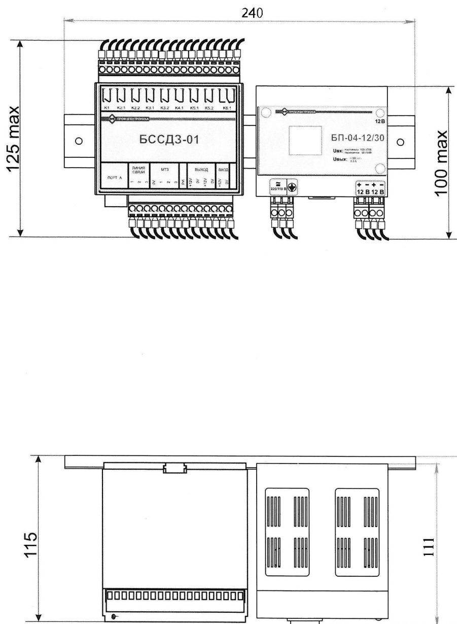
Рисунок Б.3 – Пример установки ЦМ и БП-04-12/30 на DIN-рейку
